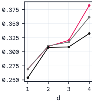
MAE (%)
